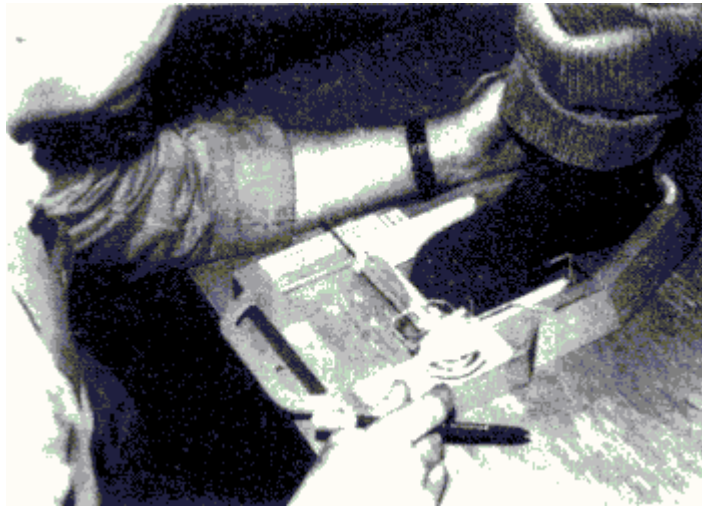
Bild 4: Vermessen des bekleideten Fußes nach Länge und größter Breite mit einem einfachen Messgerät
