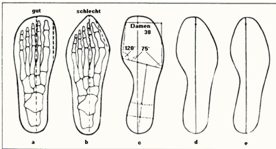
Bild 5: Brandsohlenformen
